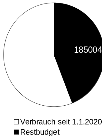
CO2 Restbudget in Tonnen für Kuppenheim
